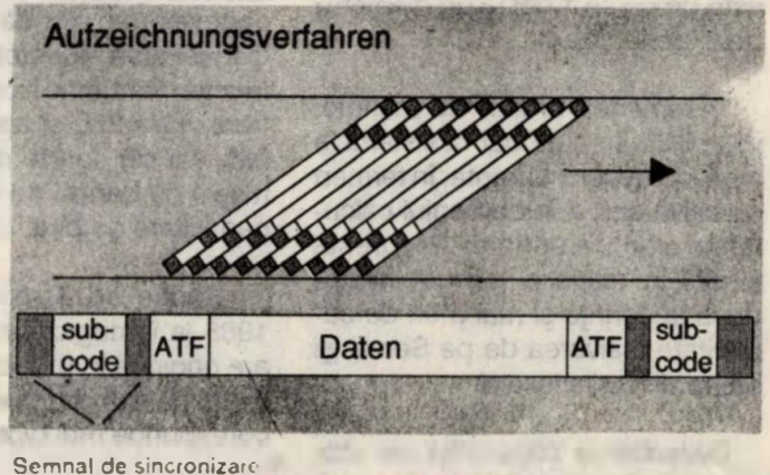
Fig. 3. Format de înregistrare pe piste oblice. Informațiile ATF și datele de corectură limitează domeniul de date.
