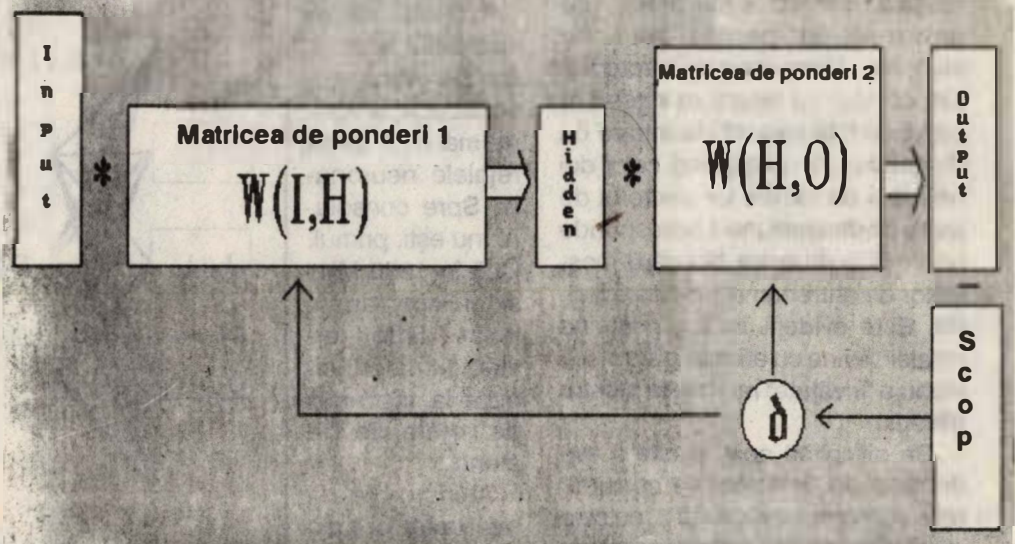
Figura 3. Vectorul de intrare determină un vector de ieșire, a cărui diferență față de vectorul scop este folosită pentru modificarea matricilor de ponderi
